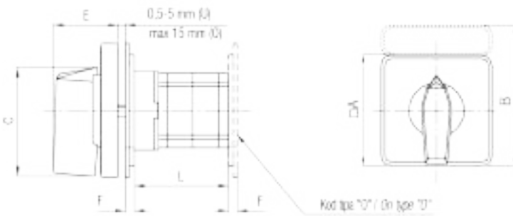
GF20H Ugradna sklopka / Front mounting (A) Sklopka za odvojenu ugradnju / Rear mounting (B)
