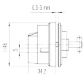
Spojka za vrata - zaključavanje lokotom - 90 Door coupling - padlock - 90
