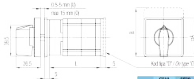
GF20 Ugradna sklopka / Front mounting (A) Sklopka za odvojenu ugradnju / Rear mounting (B)
