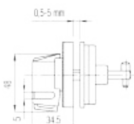
Spojka za vrata - zaključavanje lokotom - 85 Door coupling - padlock - 85
