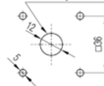
GF20 Samo na prednjoj ploči Only on the front panel
