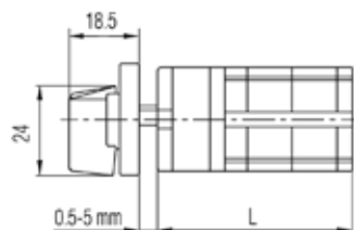
GF10 Ugradna sklopka Front mounting (U)
