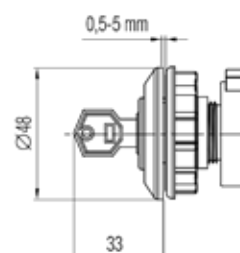
Centralna ugradnja - 29K Central mounting - 29K
