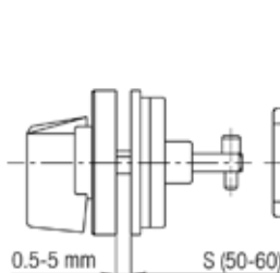
Spojka za vrata - 57/58 Door coupling - 57/58
