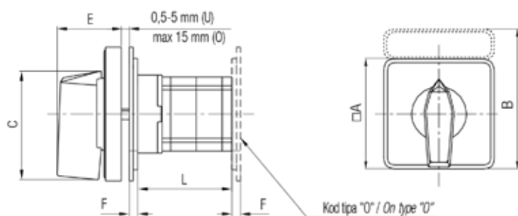
GF20H Ugradna sklopka / Front mounting (U) Sklopka za odvojenu ugradnju / Rear mounting (O)
