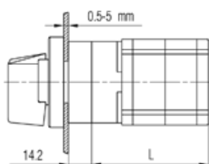
Centralna ugradnja - 20 Central mounting - 20
